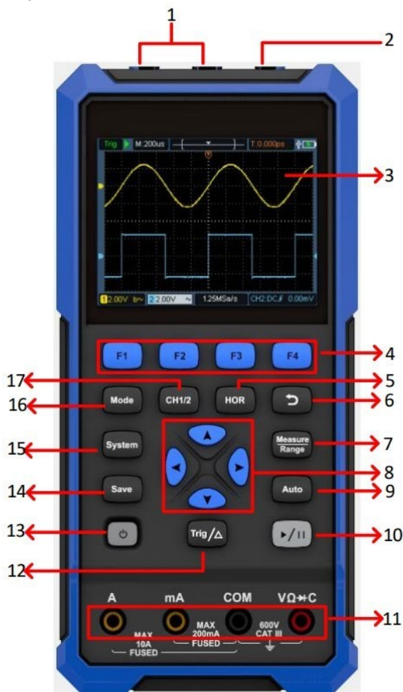
Рисунок. 3.1. Передняя панель осциллографа
