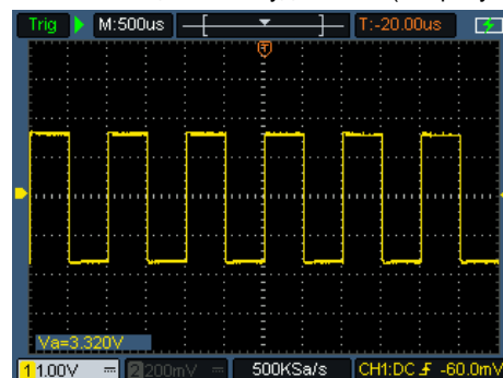
Рисунок 3.4. Автонастройка
